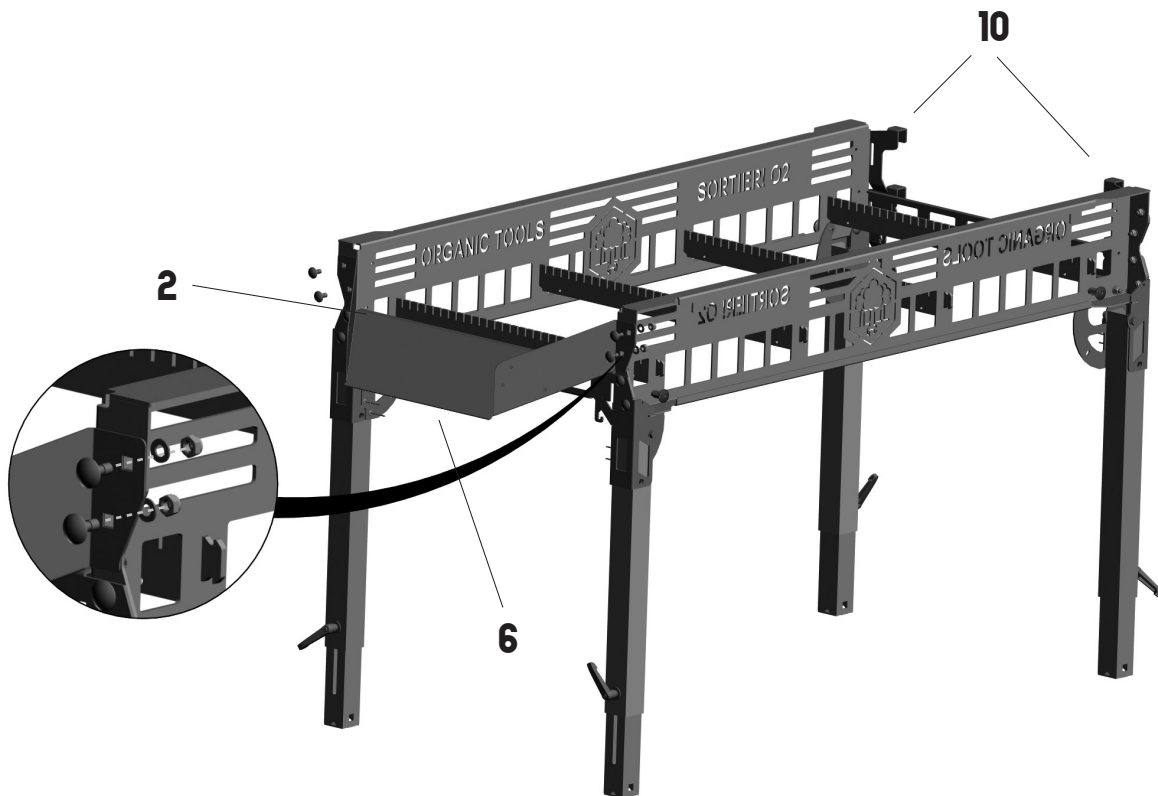
Abbildung 10: Montage des Trichters auf der Stirnseite der Seitenwangen
