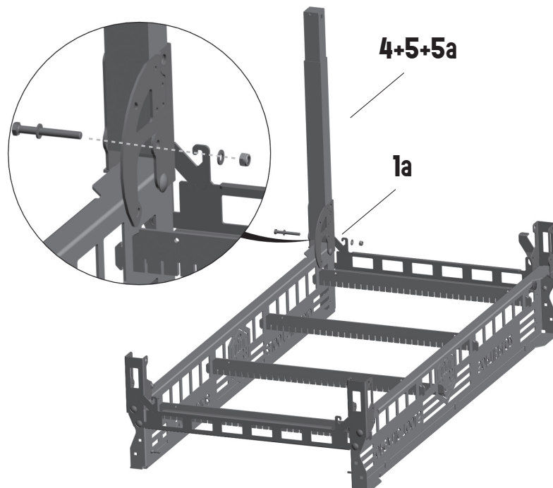
Abbildung 9: Montage der Tischbeine mit langen Sechskantschrauben von außen nach innen.
