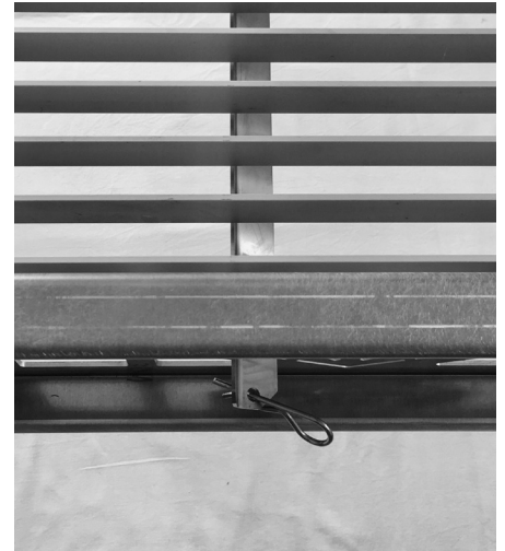
Abbildung 14: Sicherungstrebe befindet sich unter den anderen Streben
