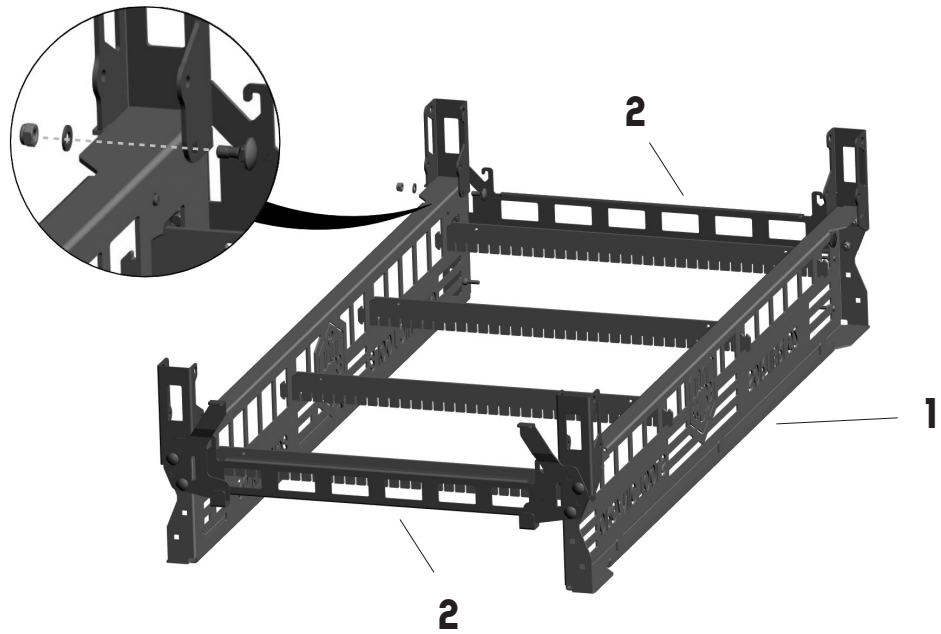
Abbildung 6: Stirnseiten (2) an Längsseite der Seitenwange (1) von innen nach außen festschrauben
