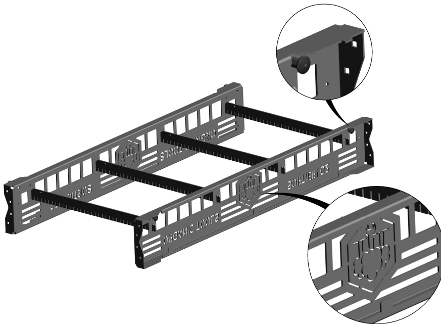
Abbildung 3: Querstreben in Seitenwangen einhängen
