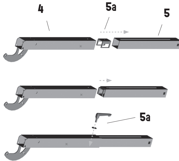
Abbildung 8: Ober- und Unterteile der Beine mit Verbindungsmitteln zusammensetzen
