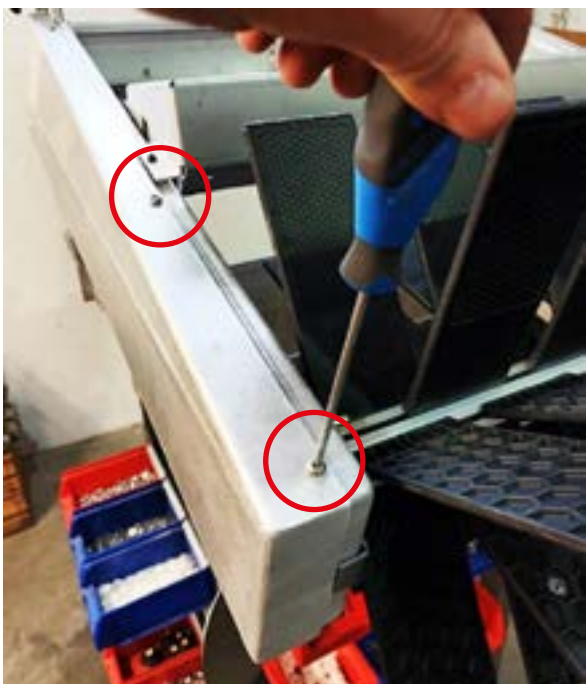
Abbildung 1: Lösen Sie die 2 vorderen Schrauben an der Oberseite der linken sowie an der rechten Seitenwange.
